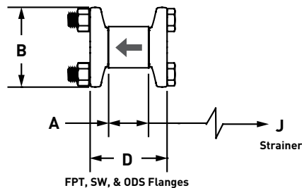
FPT, SW, &amp; ODS Flanges
