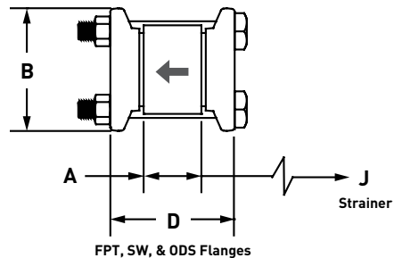
FPT, SW, &amp; ODS Flanges
